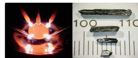
テトラアーク炉での単結晶育成とウラン化合物の単結晶 Single crystal growth in tetra-arc furnace and the single crystals of uranium compounds
