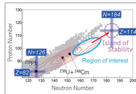
重元素および超重元素領域の核図表。安定の島の位置が示されています。等高線は、 ^{238}\text{U}+^{248}\text{Cm} の多核子移動反応で生成された原子核の収量の計算値です。Nuclei in the heavy- and superheavy-element region. The location of the Island of Stability is shown. The contour plot shows the calculated yields of nuclei produced in the ^{238}\text{U}+^{248}\text{Cm} multi-nucleon transfer reaction.
