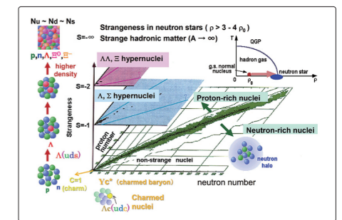
ストレンジネスを含む3次元核図表 Three dimensional nuclear chart including strangeness
