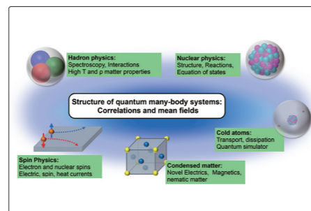
普遍的な物理を探求するグループの研究対象 Our research subjects of universal physics
